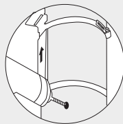
2. 브라켓 하단부 오른쪽 전선 인입부 홀 타공 (1차 3mm 스텐드릴 | 2차 8mm 스텐드릴)
