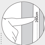
1. 가로등 2m 60cm 높이에 스텐밴드로 브라켓을 고정
